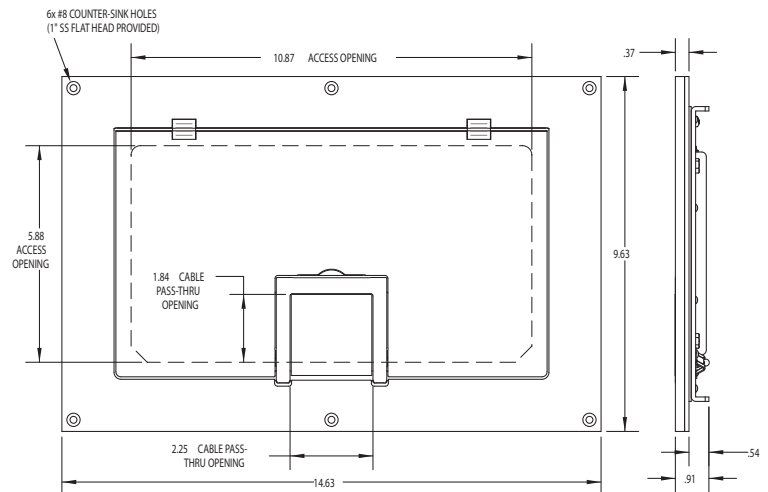
HATCH-600P-X75
